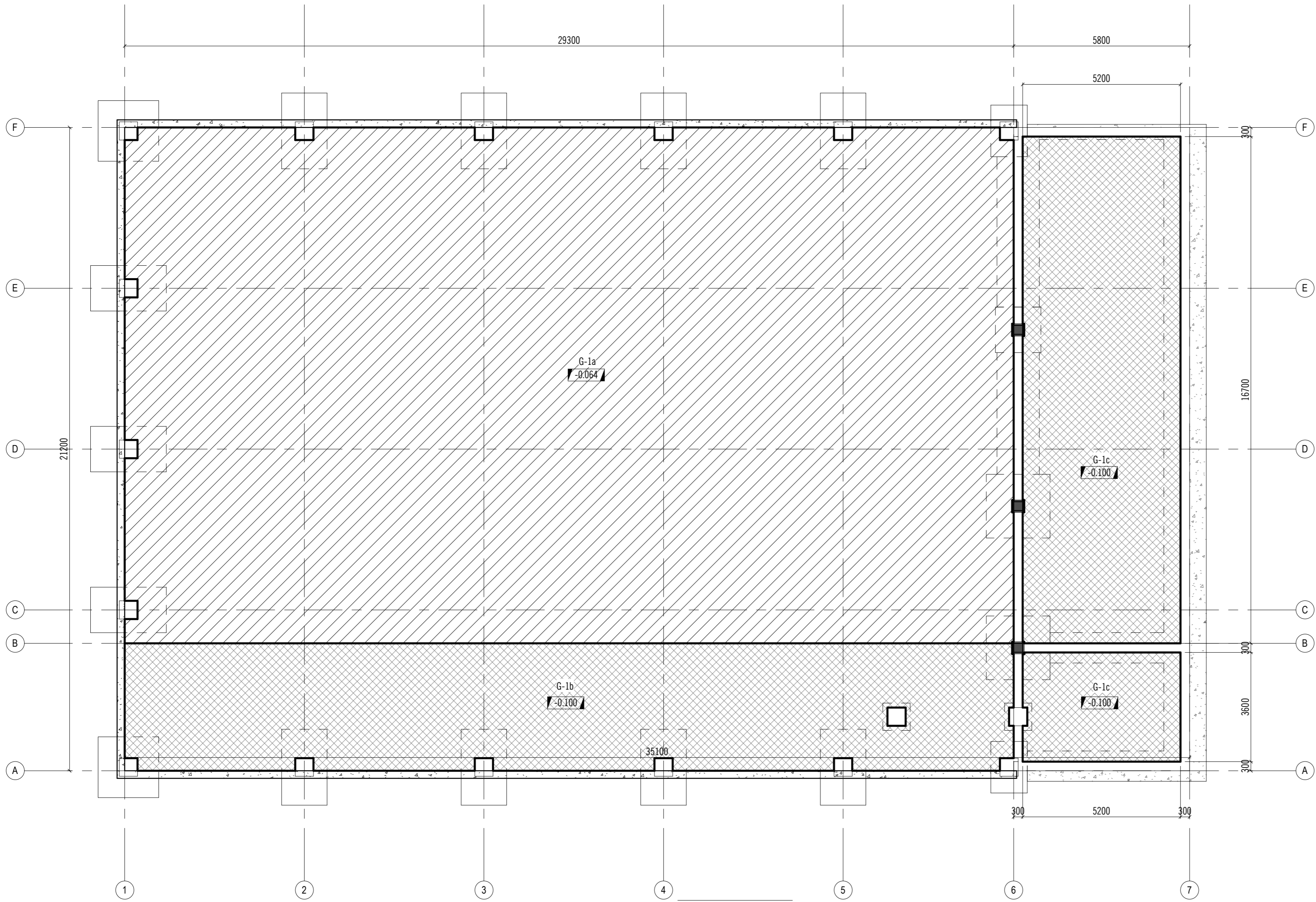
Grīda uz grunts 1 : 100
