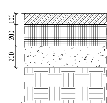
G-1b, G-1c 1 : 20
