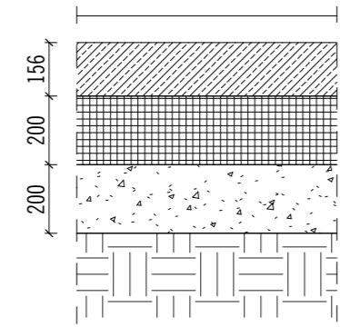
G-1a 1 : 20
